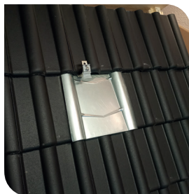
6 | Obere Dachpfanne wieder eindecken - fertig!
