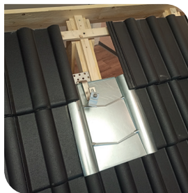
2 | Metaldachpfanne einsetzen, Dachhaken anlegen und Position markieren.
