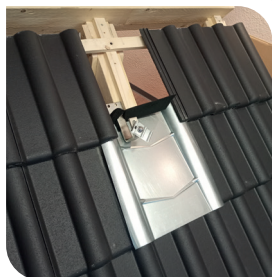
5 | Dachhaken aufschrauben.
