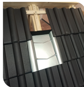
4 | Beiliegenden Schaumkeil aufkleben und für Dachhaken L-förmig ausschneiden. (*)
